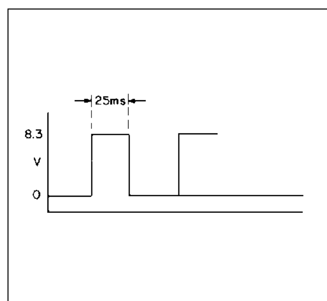
Figure 6 - SYN EN (Input To Pin 13 Of U201)
