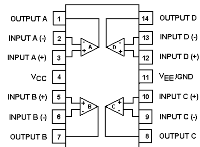
U3, U1 19A701789P4 Quad Op-Amp
