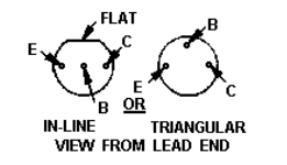
LEAD IDENTIFICATION FOR Q2, Q4, Q6-Q9, Q11, Q13-Q18
