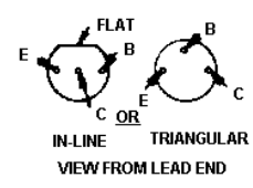
LEAD IDENTIFICATION FOR Q6, & Q9 - Q13
