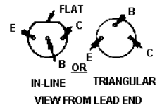
LEAD IDENTIFICATION FOR Q1 - Q5, Q7, Q8, Q14 - Q16
