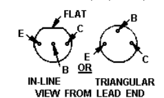
LEAD IDENTIFICATION FOR Q2, Q4, Q6-Q9, Q11, Q13-Q18
