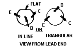
LEAD IDENTIFICATION FOR Q1 - Q5, Q7, Q8, Q14 - Q16
