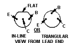
LEAD IDENTIFICATION FOR Q1, Q3, Q5, Q10, Q12
