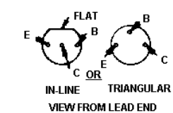
LEAD IDENTIFICATION FOR Q6, & Q9 - Q13
