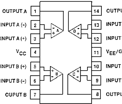
U3 19A701789P4 Quad Op-Amp
