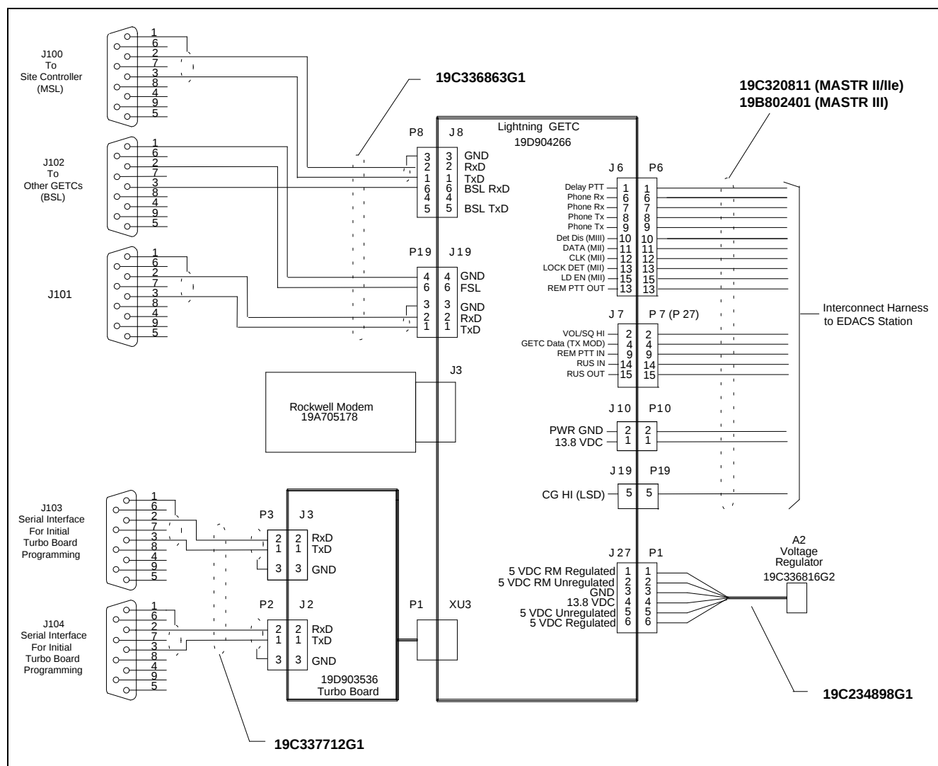
GETC CABLE 19C336863G1
