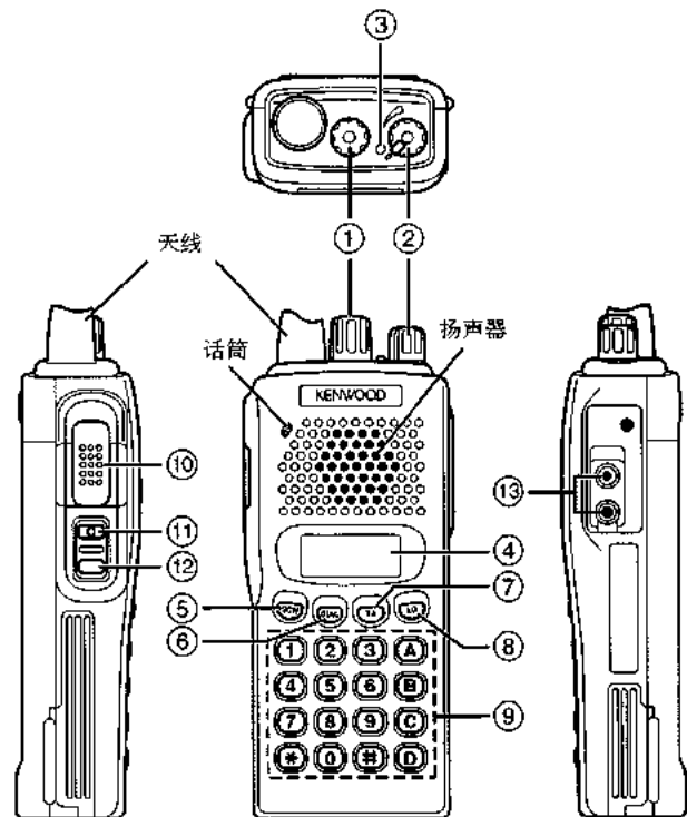
装有KNB-14电池(选件)的KNB-14的示意图
