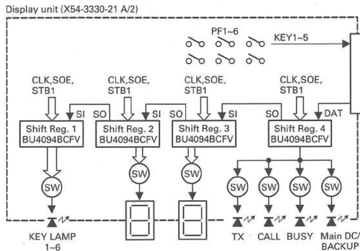
Fig. 9 Display circuit
